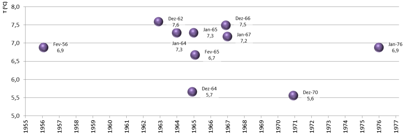
Gráfico 7 - Os 10 meses com as temperaturas mais baixas de sempre (Amadora, 1915-2012)
