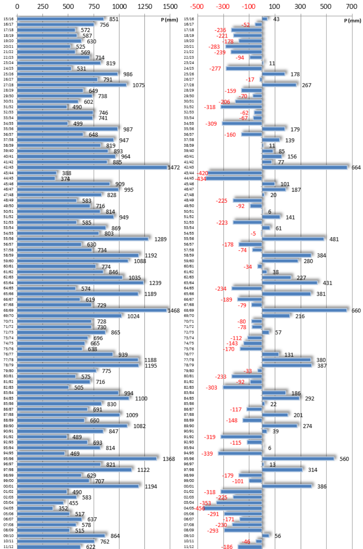
Gráfico 4 - Esquerda: precipitação média anual; Direita: desvios em relação à precipitação média anual (Amadora, 1915-2012)
