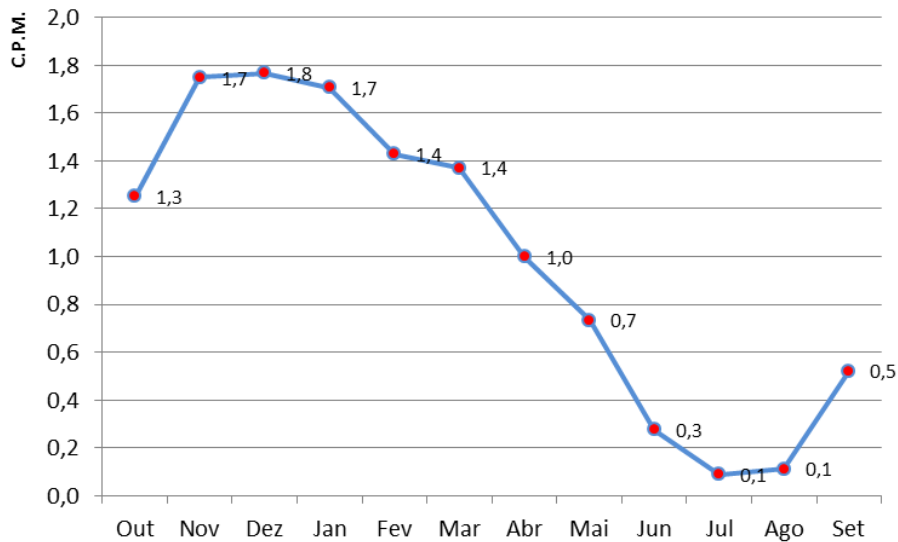
Gráfico 2 - Coeficiente pluviométrico mensal (Amadora, 1915-2012)
