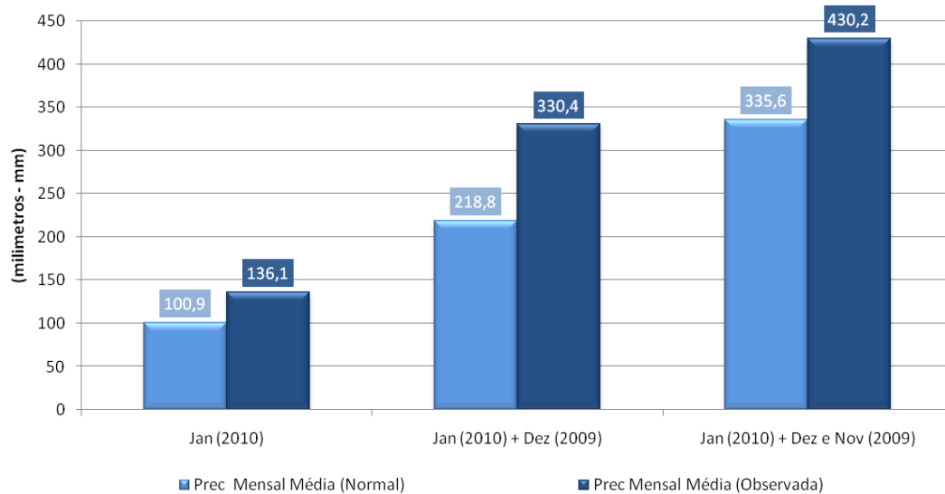
Gráfico 26 - Relação entre a precipitação média mensal (observada) e a precipitação média mensal (das normais climatológicas) nos meses de dezembro, novembro (2009) e janeiro (2010) (Amadora, 2000-2010) Dados Estatísticos: Normais Climatológicas da Amadora, 1981-2010 Tratamento e Análise Estatística: SMPC Amadora / TERCUD
