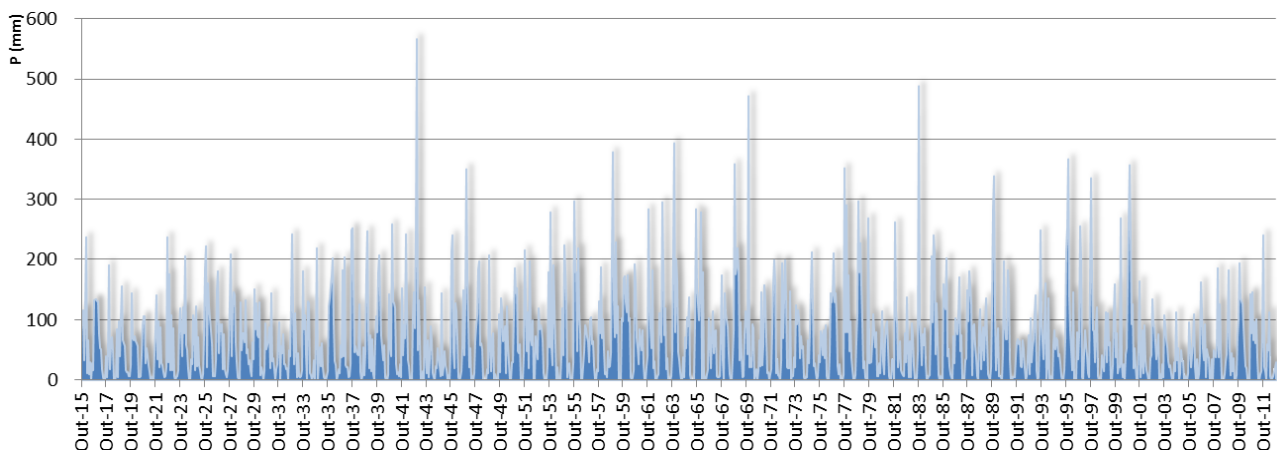
Gráfico 5 - Variação inter anual da precipitação média mensal (Amadora, 1915-2012)
