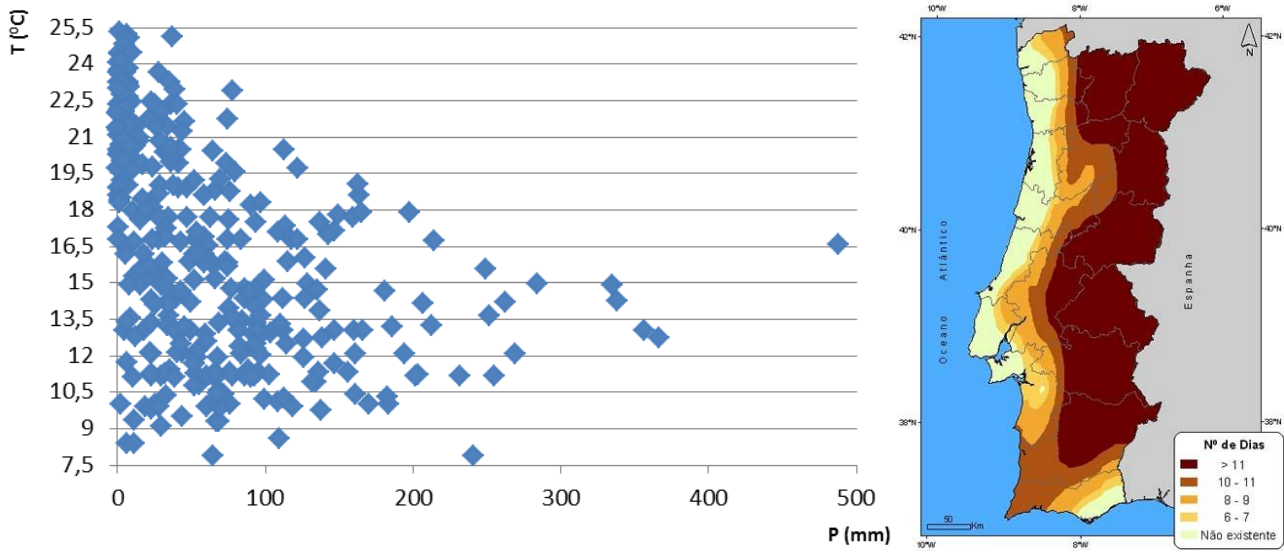
Gráfico 17 - Esquerda: precipitação e a temperatura média mensais na Amadora (Amadora, 1981-2010) Mapa 2 - Direita: duração da onda de calor de julho/agosto de 2003 18
