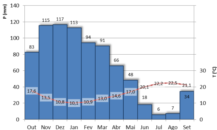
Gráfico 1 - Diagrama termopluviométrico (Amadora, 1915-2012)
