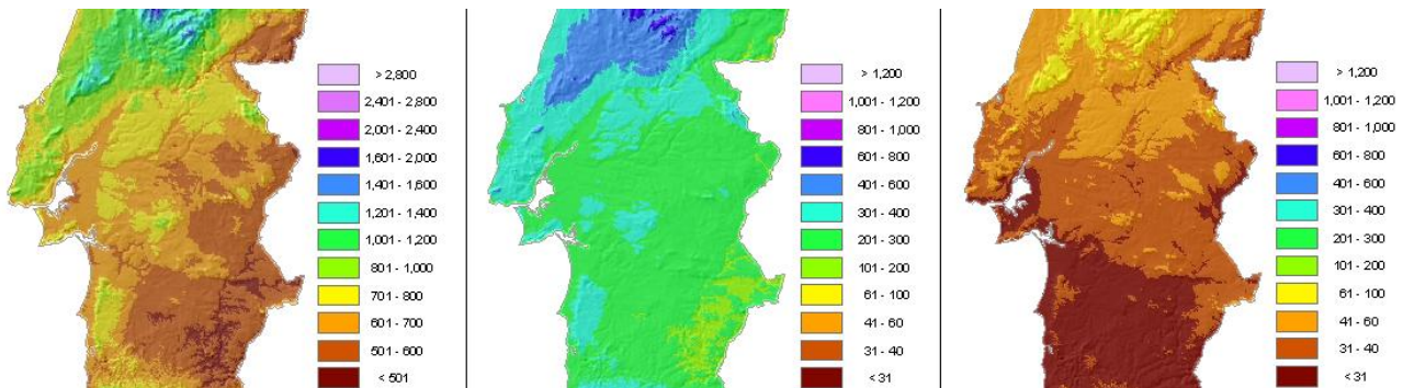
Fig. 3 - Esquerda: precipitação média anual; Centro: precipitação média no inverno; Direita: precipitação média no verão 16
