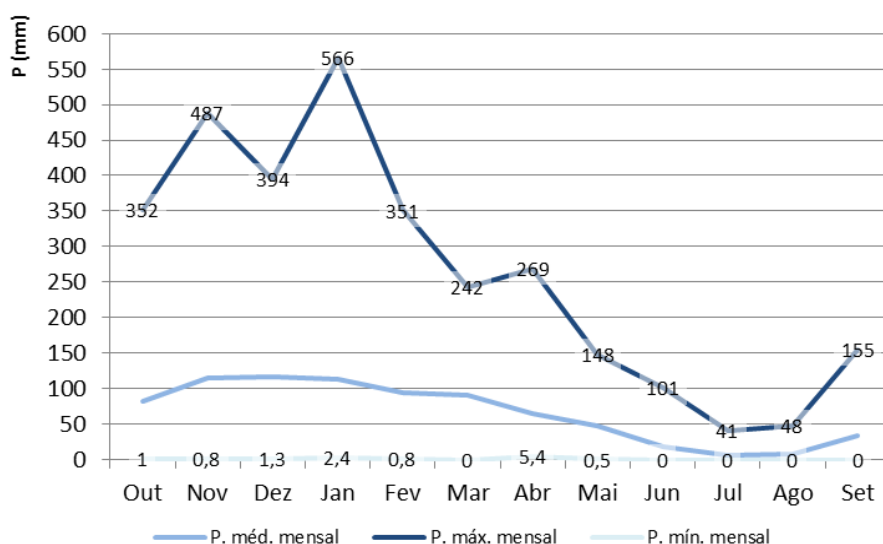
Gráfico 3 - Precipitação média, máxima média e mínima média mensais (Amadora, 1915-2012)
