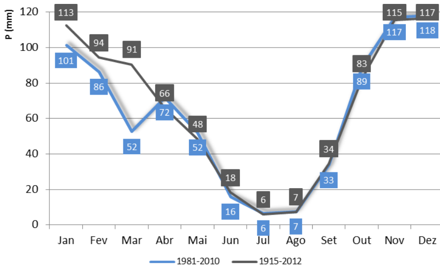
Gráfico 12 – Diferenças entre as séries de precipitação de 1981-2010 e 1915-2012 (Amadora)
