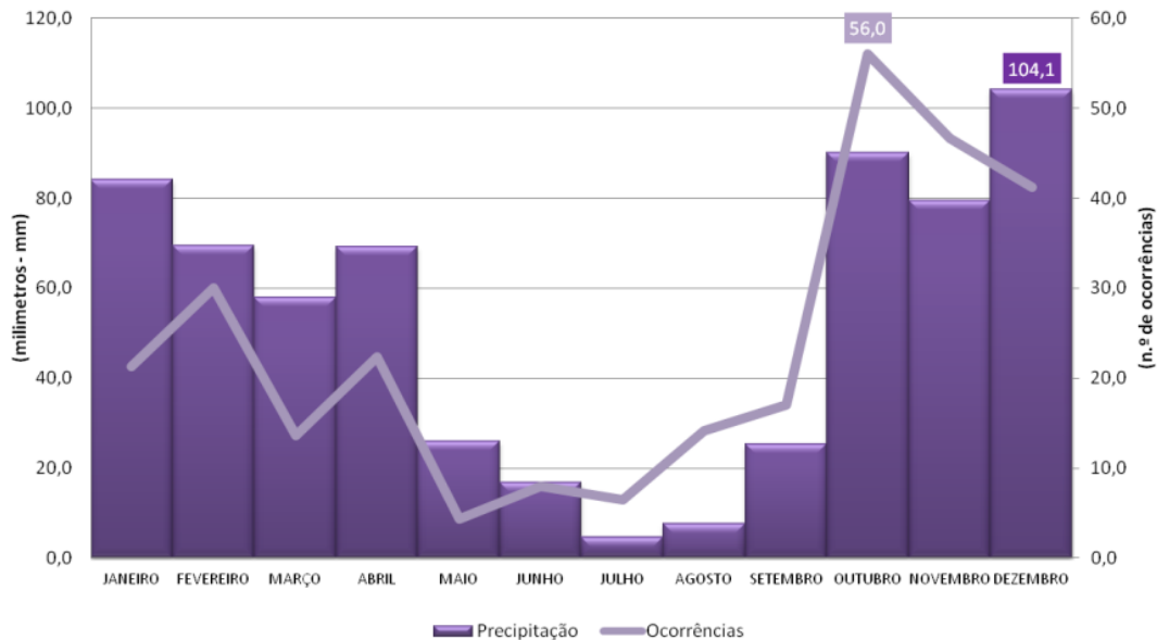
Gráfico 21 - Precipitação mensal e total de inundações urbanas (Amadora, 2000-2010) Dados Estatísticos: CDOS Lisboa e Normais Climatológicas da Amadora (1981-2010) Tratamento e Análise Estatística: SMPC Amadora / TERCUD
