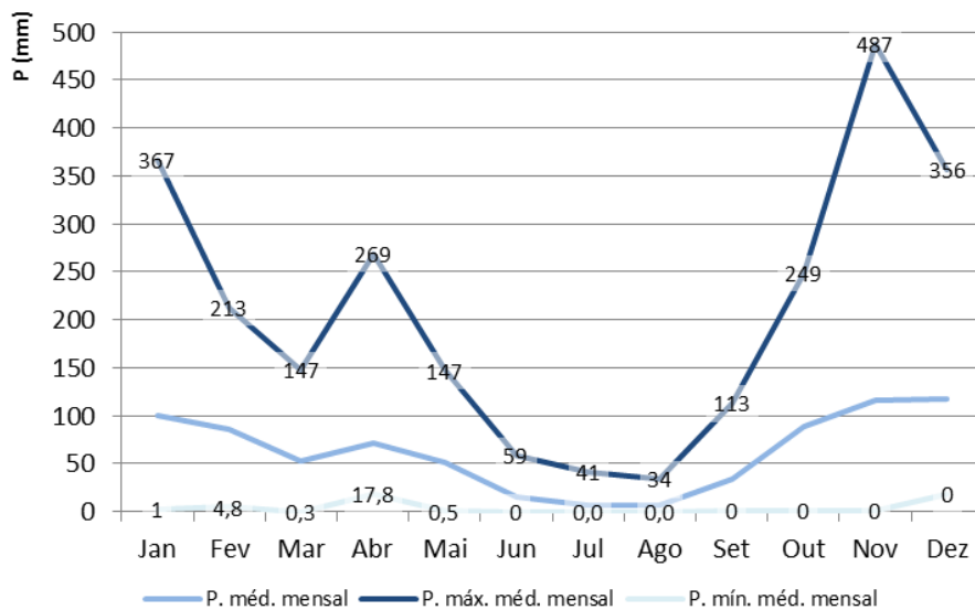
Gráfico 15 - Precipitação média, máxima média e mínima média, mensais (Amadora, 1981-2010)
